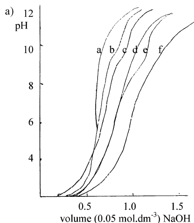
FIGURE 1 Titration curves of: (a) 0.01 \text{ mol}\cdot\text{dm}^{-3} \text{ HNO}_3 , (b) soln. (a) + 0.05 \text{ mol}\cdot\text{dm}^{-3} ligand ( L_1 ); (c) mixture (b) + 0.001 \text{ mol}\cdot\text{dm}^{-3} \text{ Cr(III)} ; (d) soln. (a) + 0.05 \text{ mol}\cdot\text{dm}^{-3} ligand ( L_2 ); (e) mix. (d) + 0.001 \text{ mol}\cdot\text{dm}^{-3} \text{ Cr(III)} ; (f) mixture (e) + 0.05 \text{ mol}\cdot\text{dm}^{-3} ligand ( L_1 ); t = 25^\circ\text{C} , \mu = 0.1 \text{ mol}\cdot\text{dm}^{-3} \text{ NaNO}_3 .
